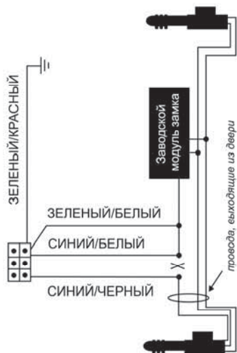
Схема 5. Однопроводный тип цепи дверных замков с оприцательной полярностью (некоторые автомобили марки Ниссан, Mazda и др.)
